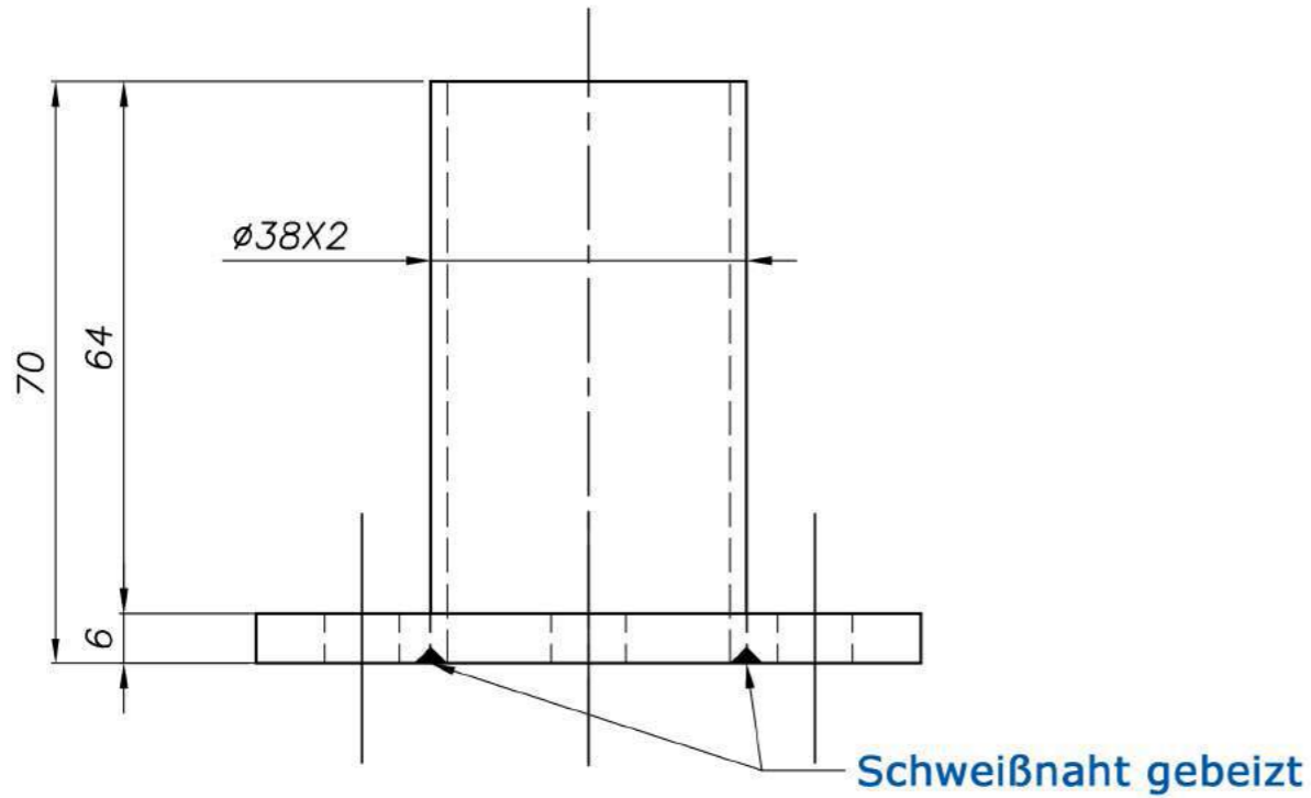
Frontalansicht
