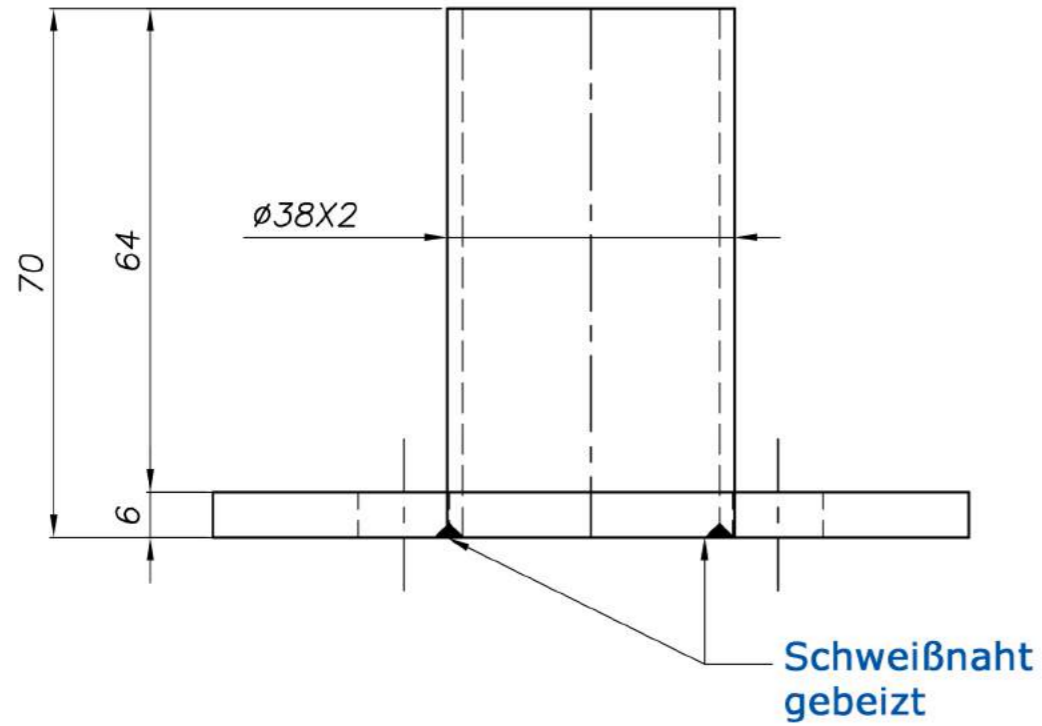
Vorderansicht
