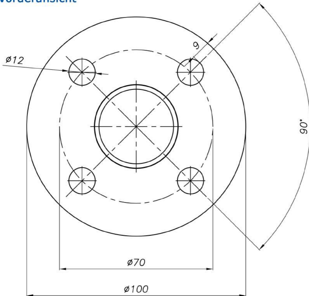
Vorderansicht
