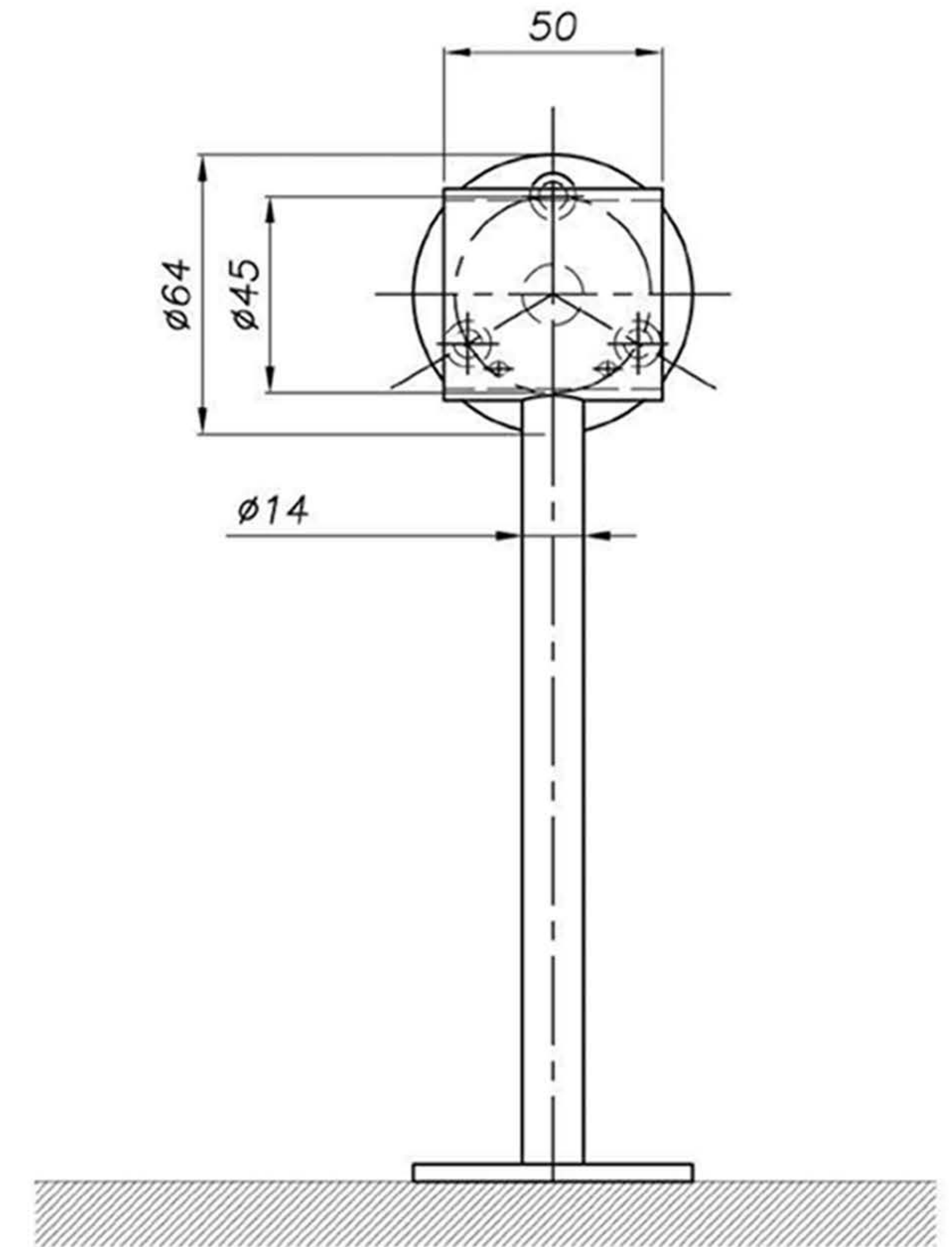
Vorderansicht
