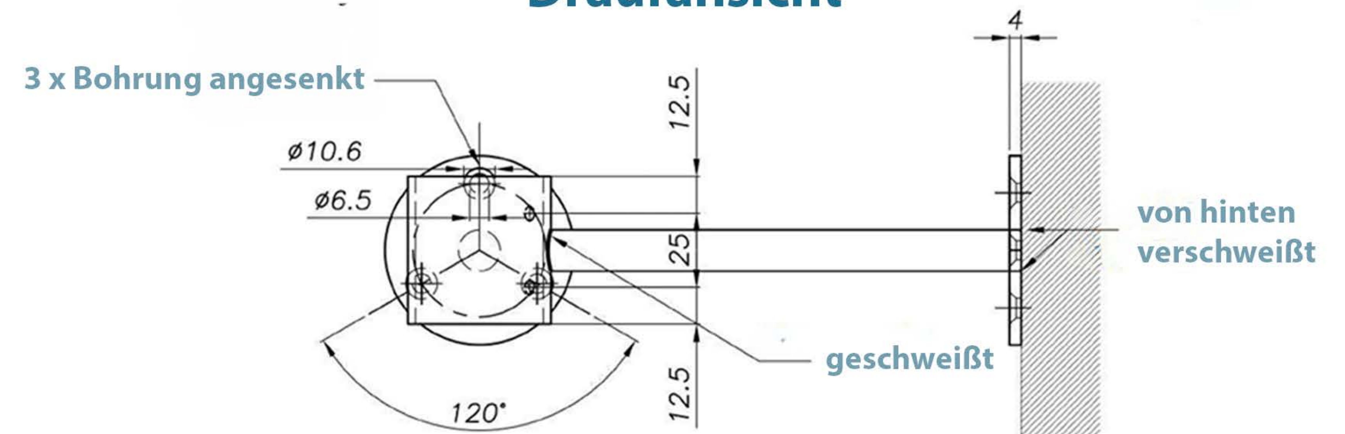
Draufansicht
