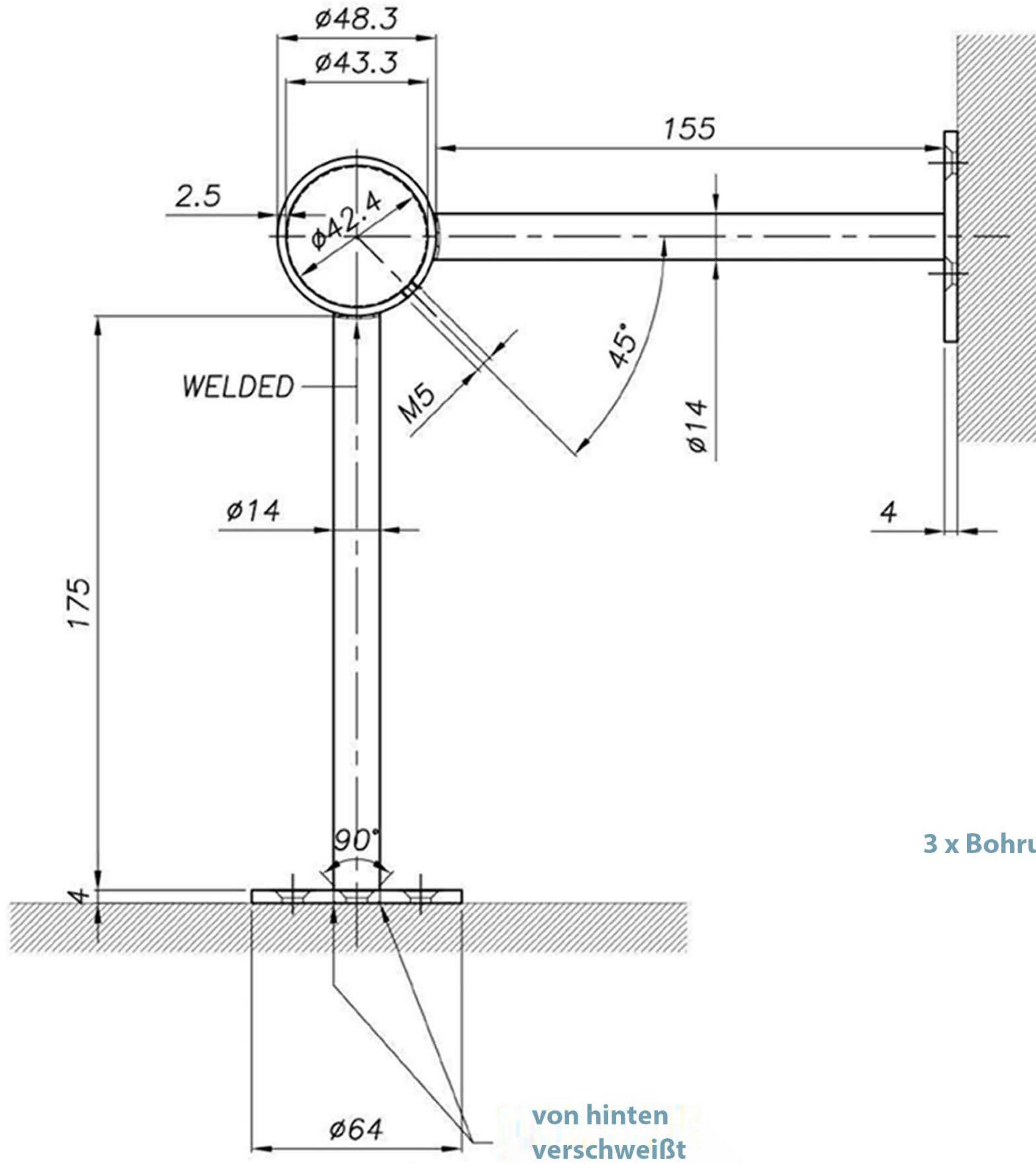
Seitenansicht
